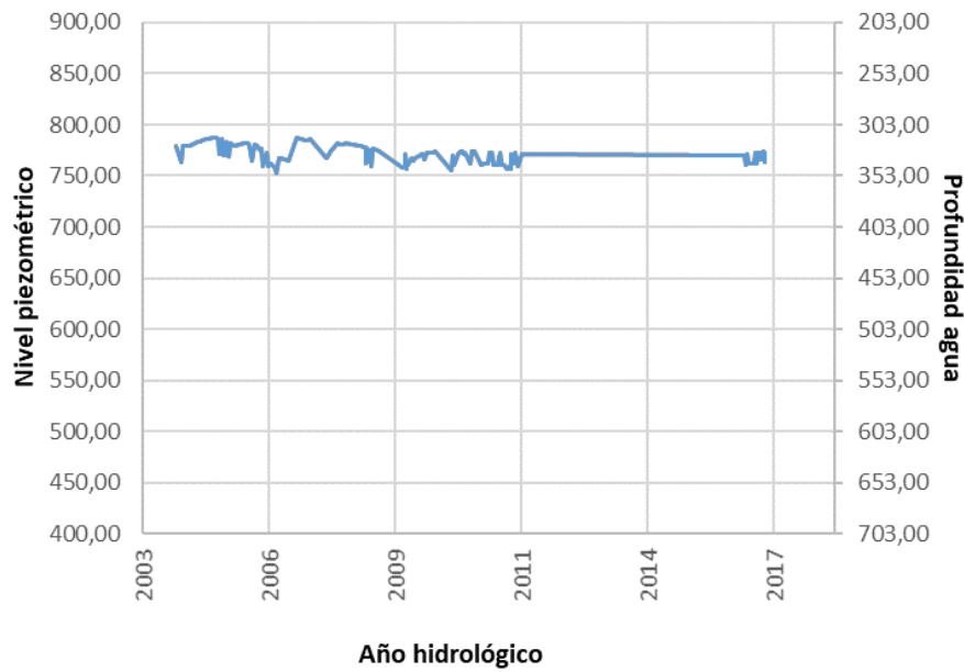
Figura 3. Evolución del nivel piezométrico y la profundidad del agua en el sondeo de Palomas II (Ac. Insular ES70LG001).
