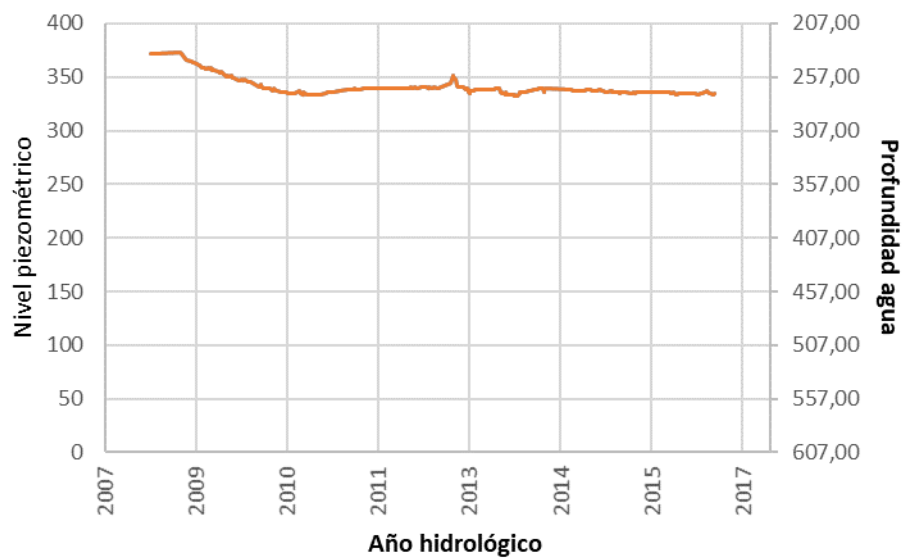
Figura 6. Evolución del nivel piezométrico y la profundidad del agua en el sondeo de Enchereda II (Ac. Insular ES70LG001).
