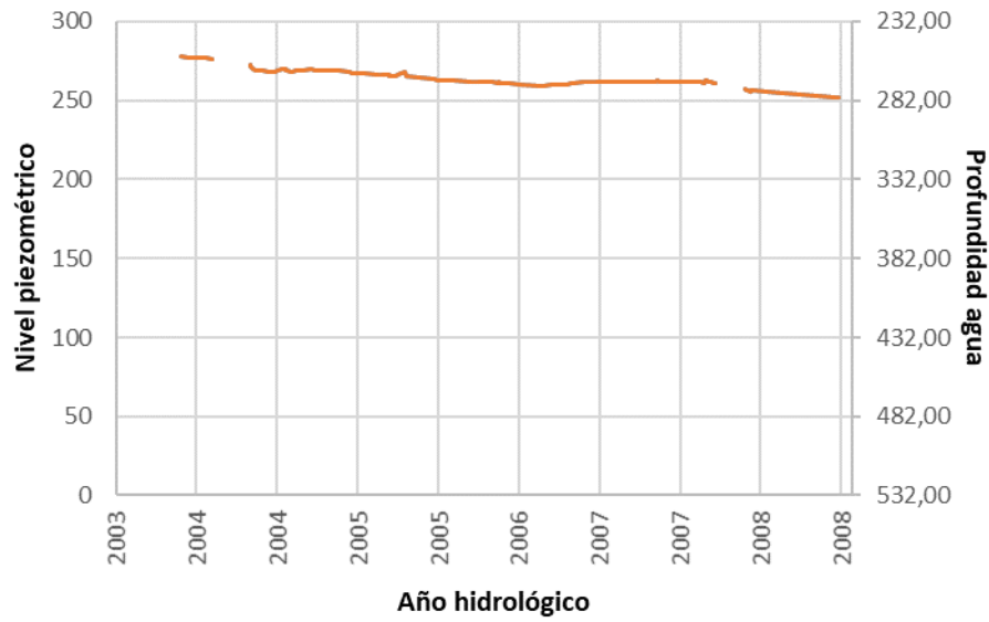
Figura 5. Evolución del nivel piezométrico y la profundidad del agua en el sondeo de Enchereda I (Ac. Insular ES70LG001).
