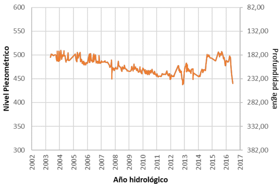
Figura 11. Evolución del nivel piezométrico y la profundidad del agua en el sondeo de Juel (Ac. Insular ES70LG001).
