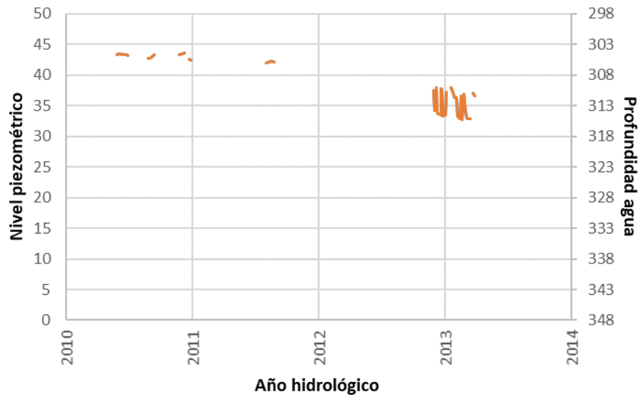
Figura 9. Evolución del nivel piezométrico y la profundidad del agua en el sondeo de La Hurona II (Ac. Costero ES70LG002).
