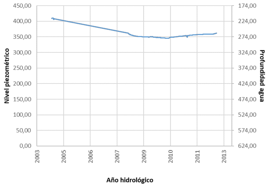
Figura 7. Evolución del nivel piezométrico y la profundidad del agua en el sondeo de Ventana Diablo (Ac. Insular ES70LG001).
