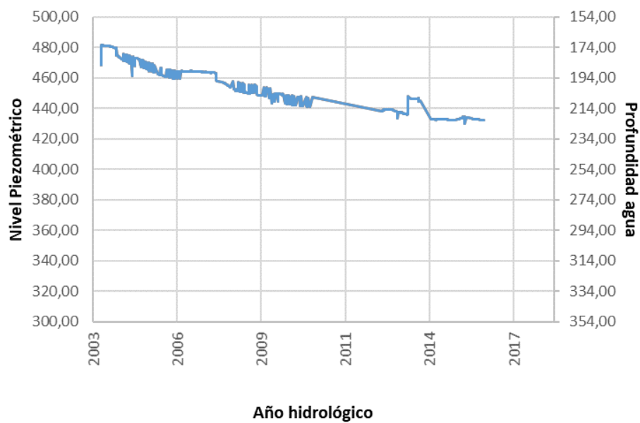
Figura 10. Evolución del nivel piezométrico y la profundidad del agua en el sondeo de Los Campos (Ac. Insular ES70LG001).
