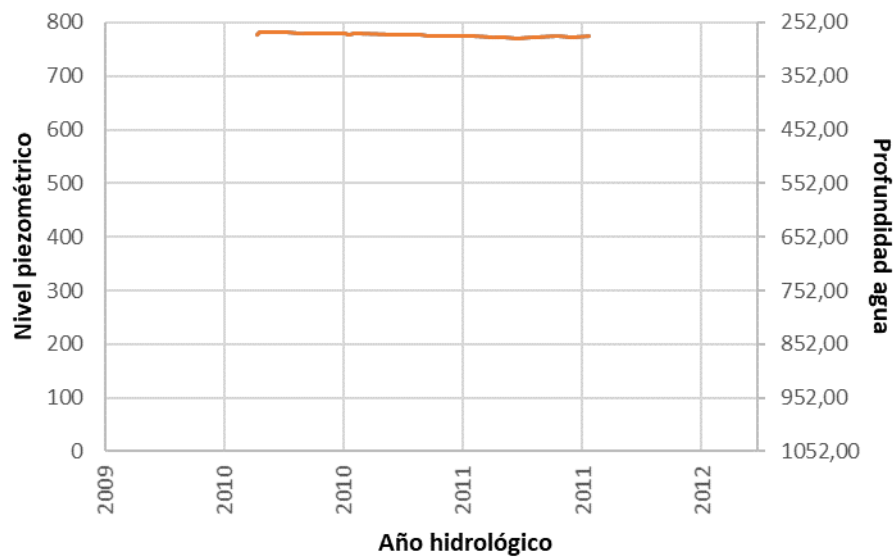
Figura 4. Evolución del nivel piezométrico y la profundidad del agua en el sondeo de Palomas IV (Ac. Insular ES70LG001).
