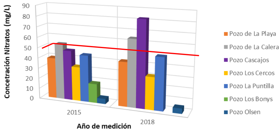
Figura 1. Evolución de las concentraciones de nitratos (mg/l) en el periodo de seguimiento (2015-2018). La línea roja muestra el límite de concentración admisible asociada a nitratos.
